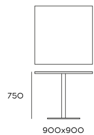
Tavolo quadrato square table, quadratischer Tisch
