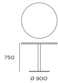
Tavolo tondo round table, rund Tisch
